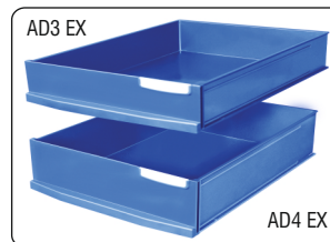
INTERNAL SIZE OF DRAWERS AD3 EX : 360mm (D) x 270mm (W) x 62mm (H) AD4 EX : 360mm (D) x 270mm (W) x 87mm (H)
