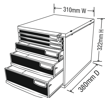
INTERNAL SIZE OF DRAWERS AD3 EX : 360mm (D) x 270mm (W) x 62mm (H) AD4 EX : 360mm (D) x 270mm (W) x 87mm (H)
