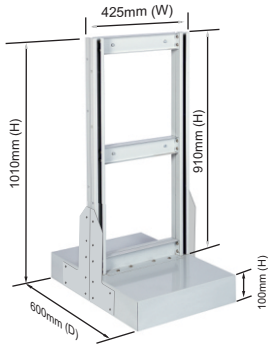
Double Sided Base Unit Stand 425 (W) x 1010 (H) x 600 (D)mm
