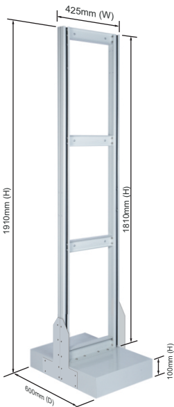
Double Sided Base Unit Stand 425 (W) x 1910 (H) x 600 (D)mm
