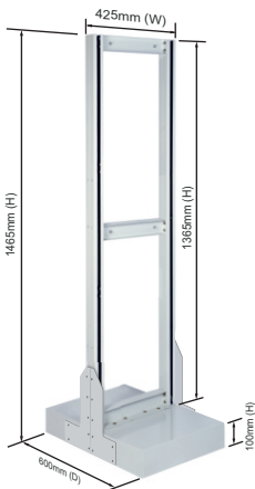
Double Sided Base Unit Stand 425 (W) x 1465 (H) x 600 (D)mm
