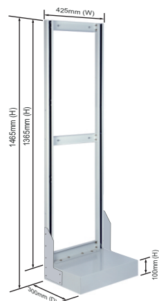
Single Sided Base Unit Stand 425 (W) x 1465 (H) x 300 (D)mm
