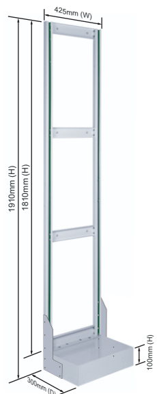
Single Sided Base Unit Stand 425 (W) x 1910 (H) x 300 (D)mm
